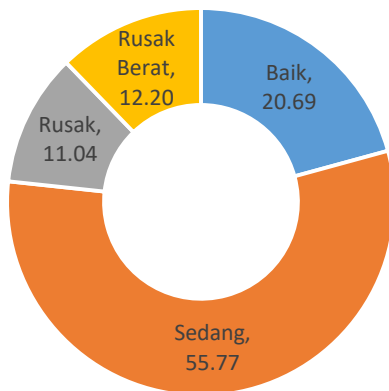
Grafik 12. Persentase Kondisi Jalan di Kabupaten Tanjung Jabung Timur, 2020
